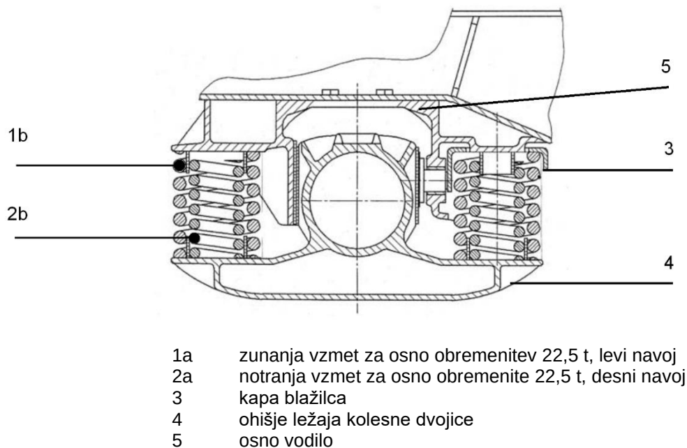
Slika 2 – Podstavni voziček s kompletom vzmeti za osno obremenitev 22,5 t
