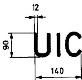
Slika 2 Znak za unificirane vagone
